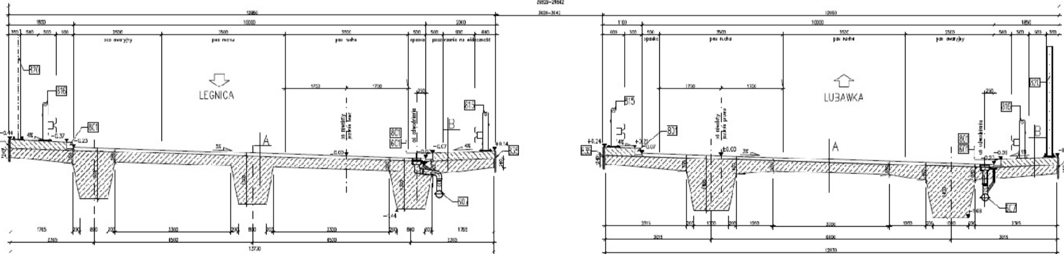
PRZEKRÓJ POPRZECZNY PRZESŁOWNY, NORMALNY 1:50
