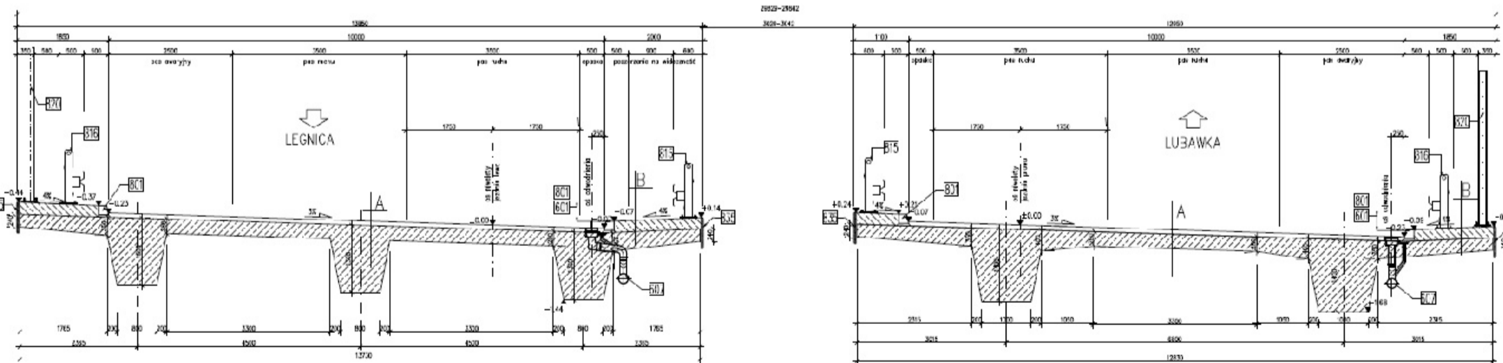
PRZEKRÓJ POPRZECZNY PRZESŁOWY, NORMATYWNY 1:30
